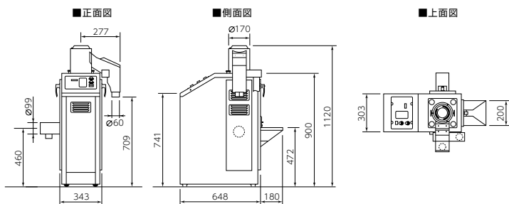
KMS-37/寸法図(mm)
