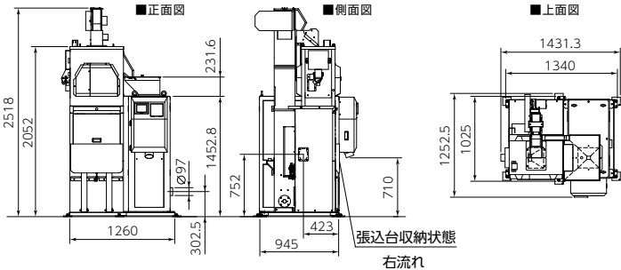
MPCA-100/寸法図(mm)
