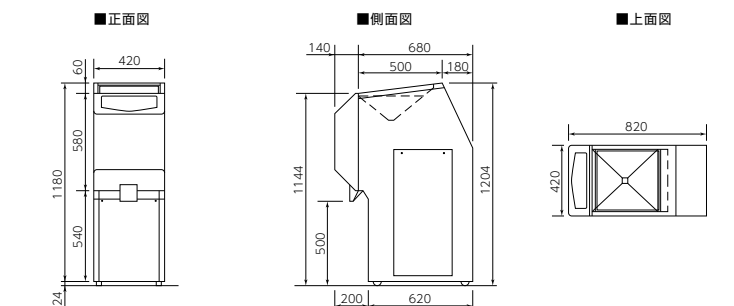
CA-50/寸法図(mm)
