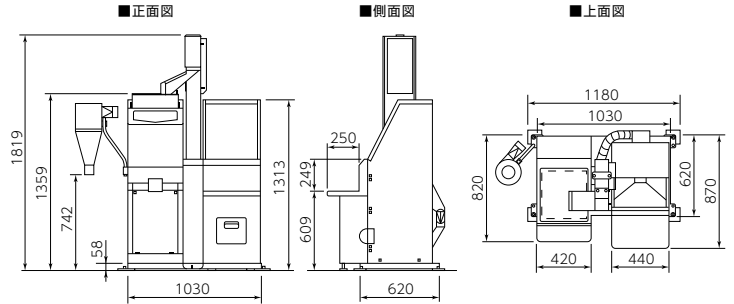
MPCA-50/寸法図(mm)
