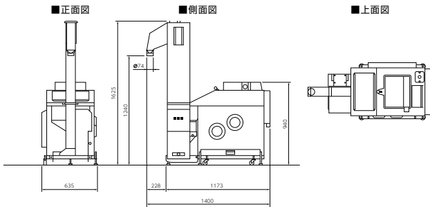
TS-2200E/寸法図(mm)
